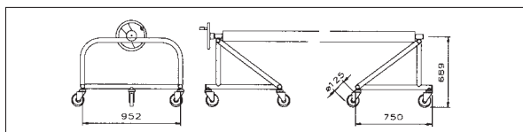
Подвижни подпори с 1 прът. Размери в mm, in mm.
