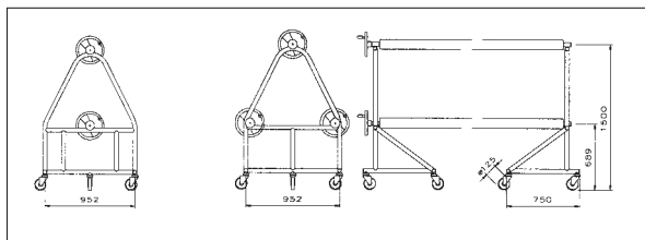
Подвижни подпори с 2 и 3 пръта. Размери в mm.
